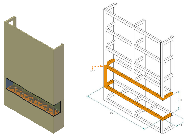
Tweezijdige montage
